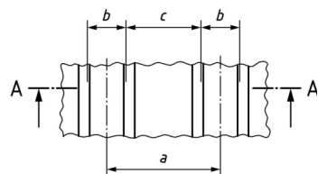
Ryc. 6.7. Faktura kierunkowa (typ A) Wymiary wypustek na podstawie normy DIN 32984: a = 37-39 \text{ mm} b = 9-11 \text{ mm} c = 27-29 \text{ mm} h = 4,5-5 \text{ mm} (przy tolerancji 0,5 mm) i zawsze h \geq 4,5 \text{ mm}
