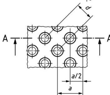
Ryc. 6.8. Faktura bezpieczeństwa (typ B). Wymiary wypustek na podstawie normy DIN 32984: a = 58-60 \text{ mm} b = 20-22 \text{ mm} c = 37-39 \text{ mm} d = 40-42 \text{ mm} h = 4,5-5 \text{ mm} (przy tolerancji 0,5 mm) i zawsze h \geq 4,5 \text{ mm}
