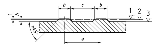
Ryc. 6.7. Faktura kierunkowa (typ A) Wymiary wypustek na podstawie normy DIN 32984: a = 37-39 \text{ mm} b = 9-11 \text{ mm} c = 27-29 \text{ mm} h = 4,5-5 \text{ mm} (przy tolerancji 0,5 mm) i zawsze h \geq 4,5 \text{ mm}
