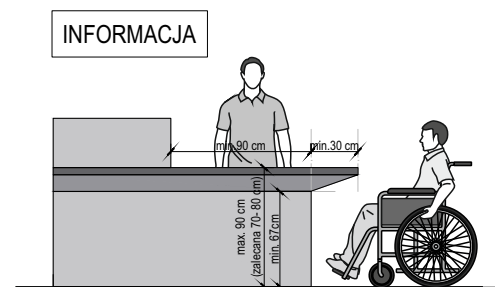
Ryc. 2.6. Lada punktu informacji (oprac. autora)
